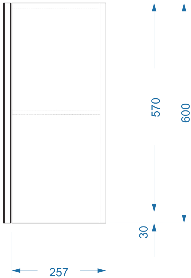
boční pohled
